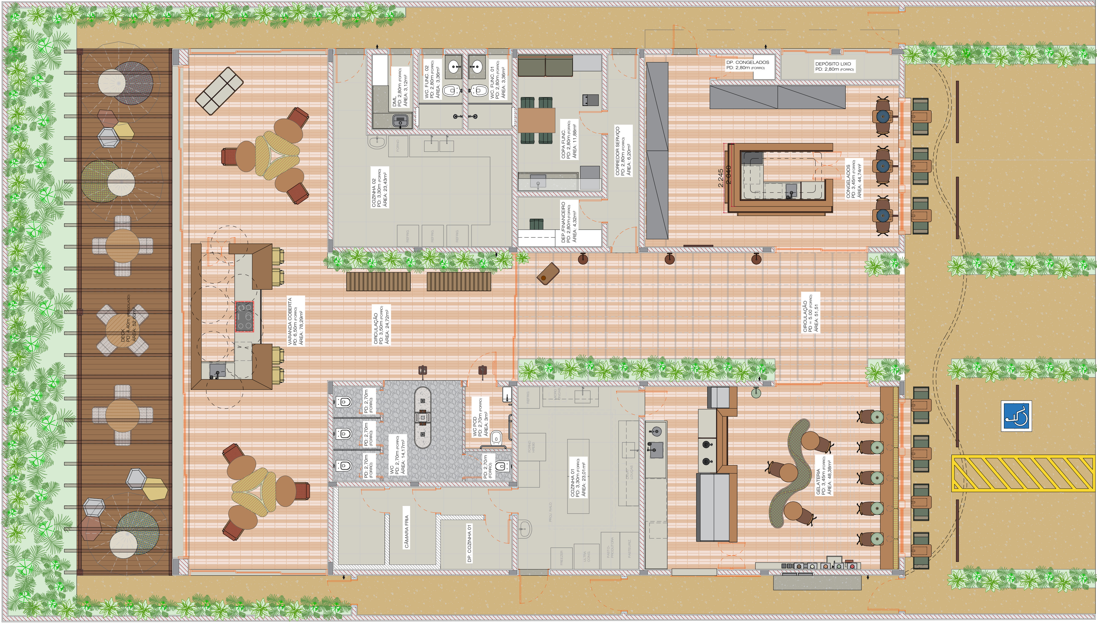
PLANTA BAIXA esc 1:75
