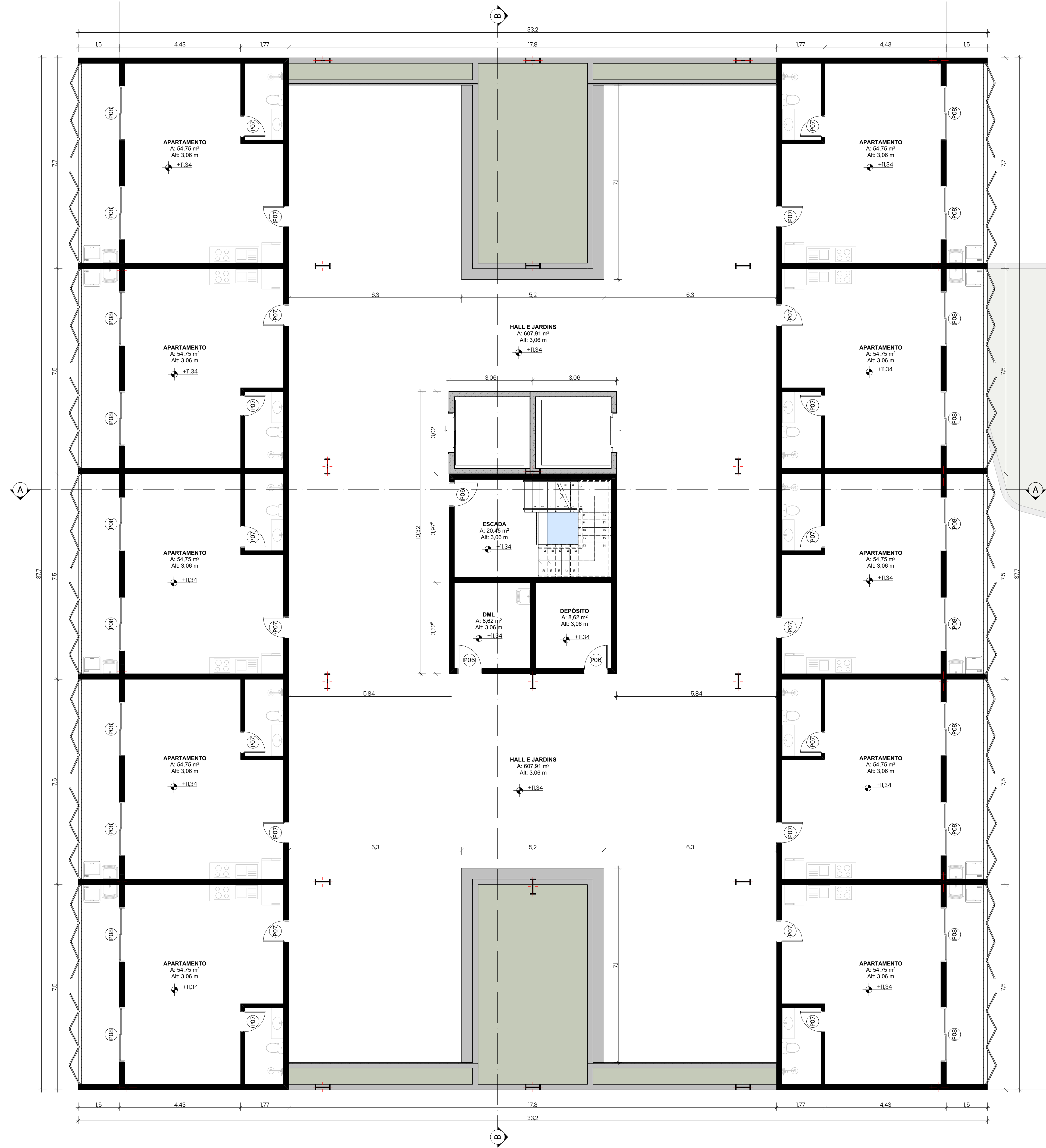
Planta Baixa - Quarto Pavimento (Pav. Tipo 1)
