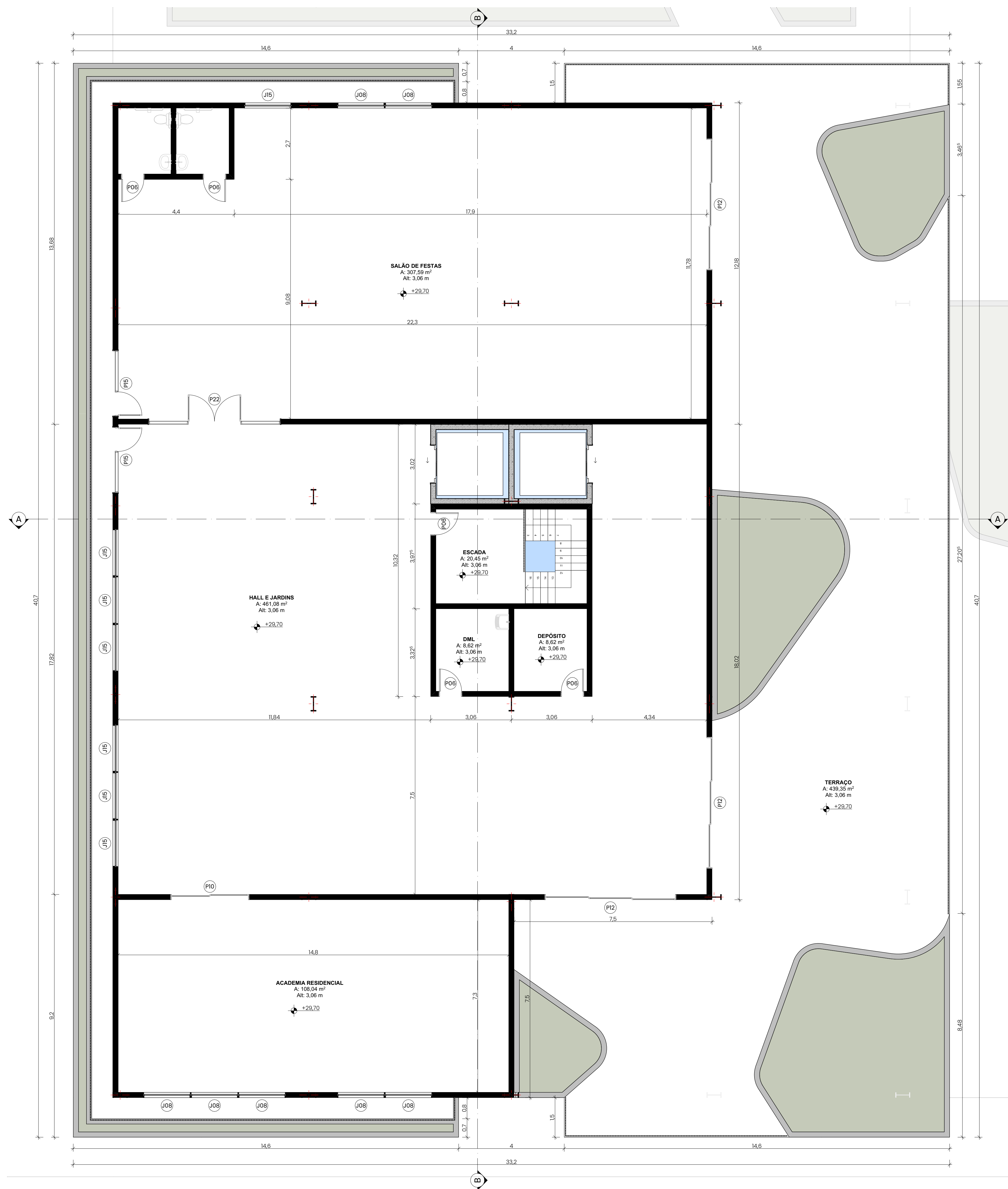
Planta Baixa - Décimo Pavimento 1:75
