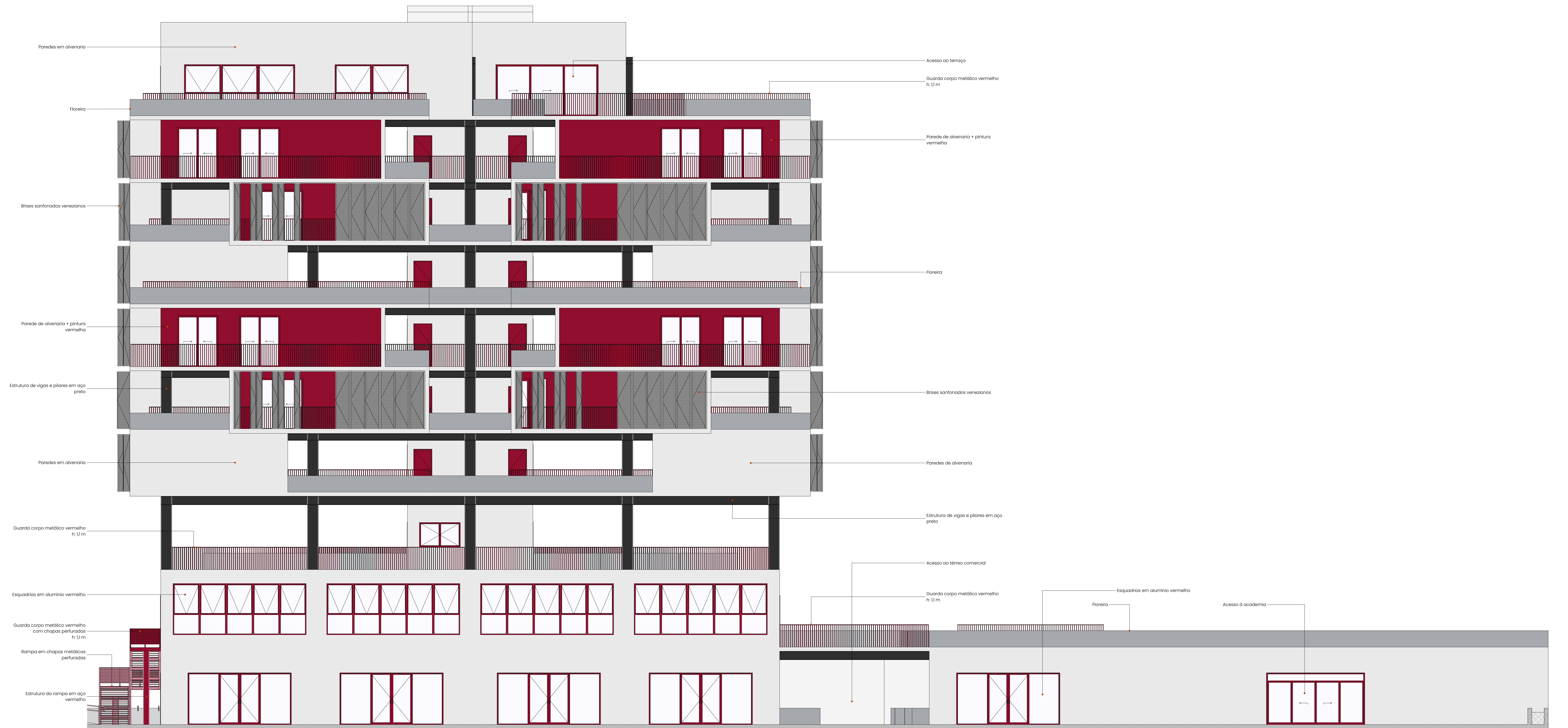
Fachada Lateral Direita 1:75
