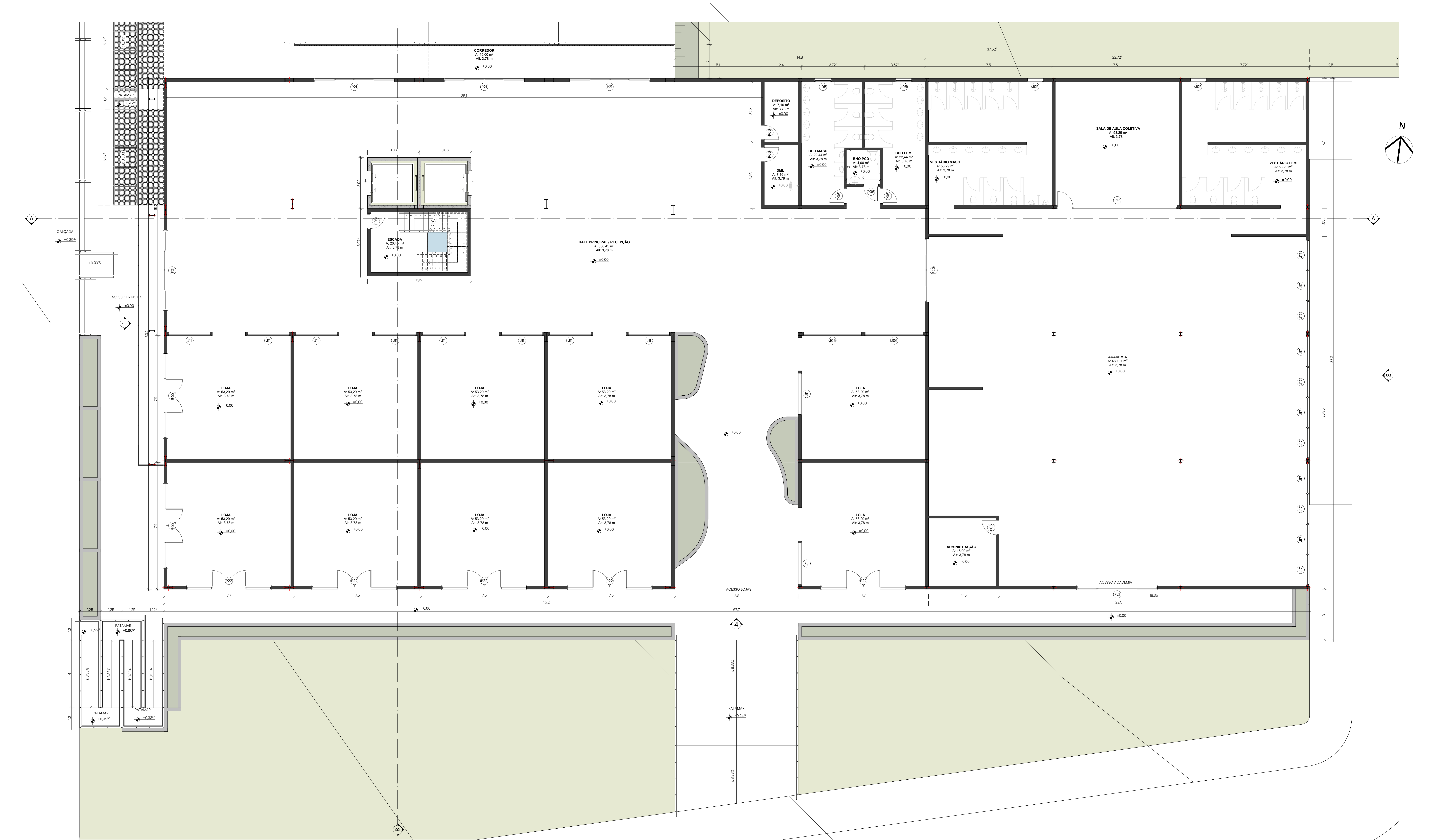
Planta Baixa – Pavimento Térreo 1:75
