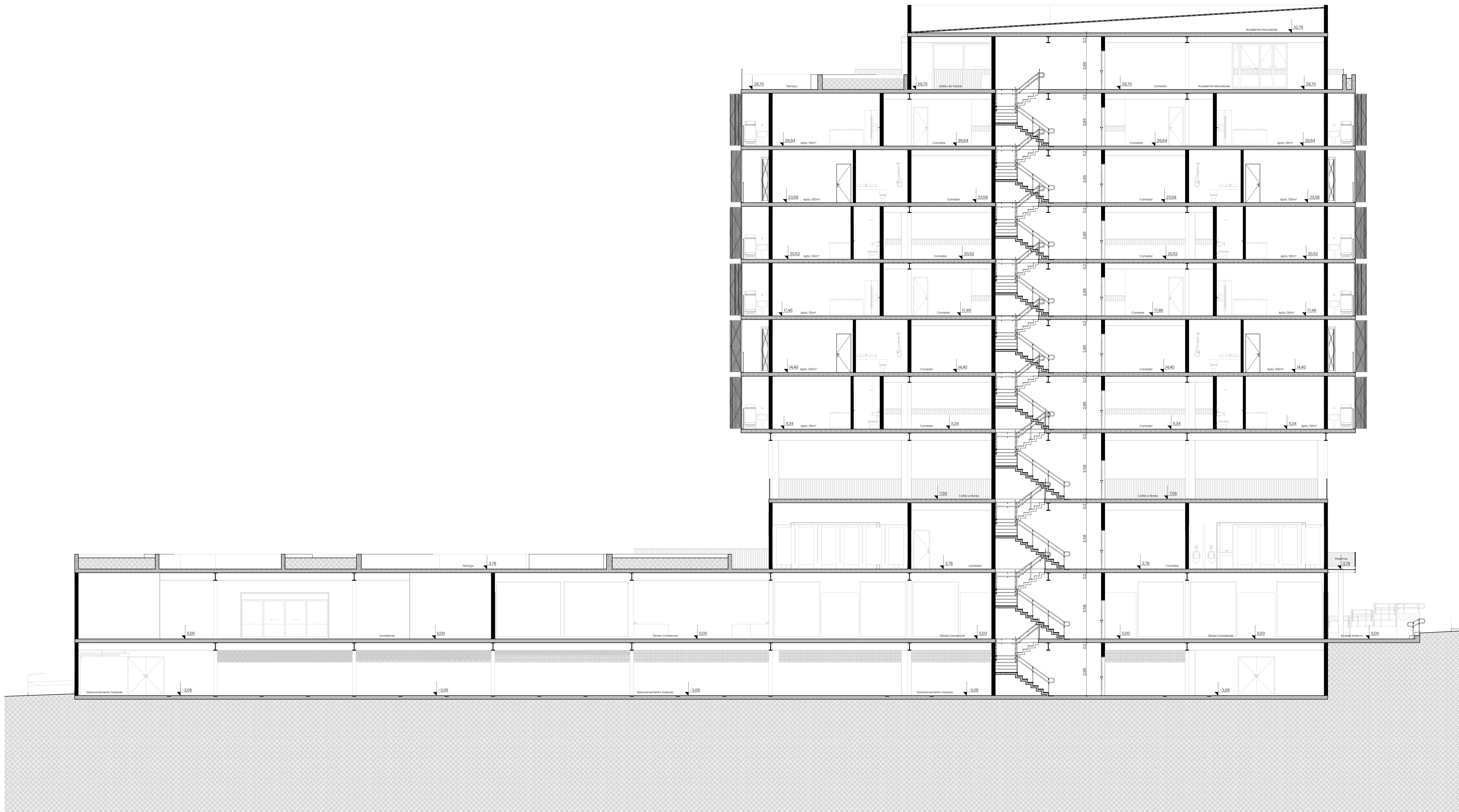
Corte AA 1:75
