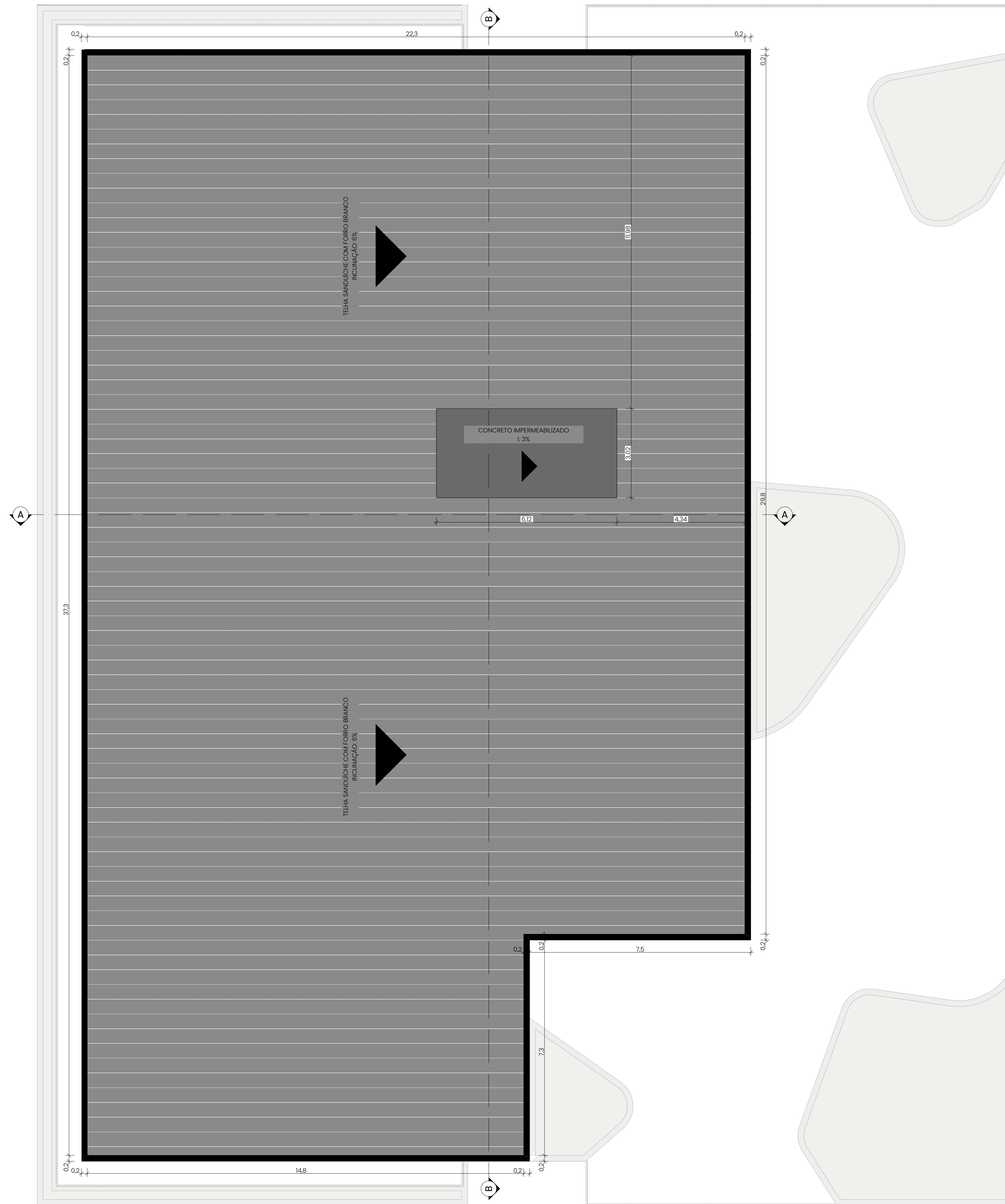
Planta de Cobertura 1:75
