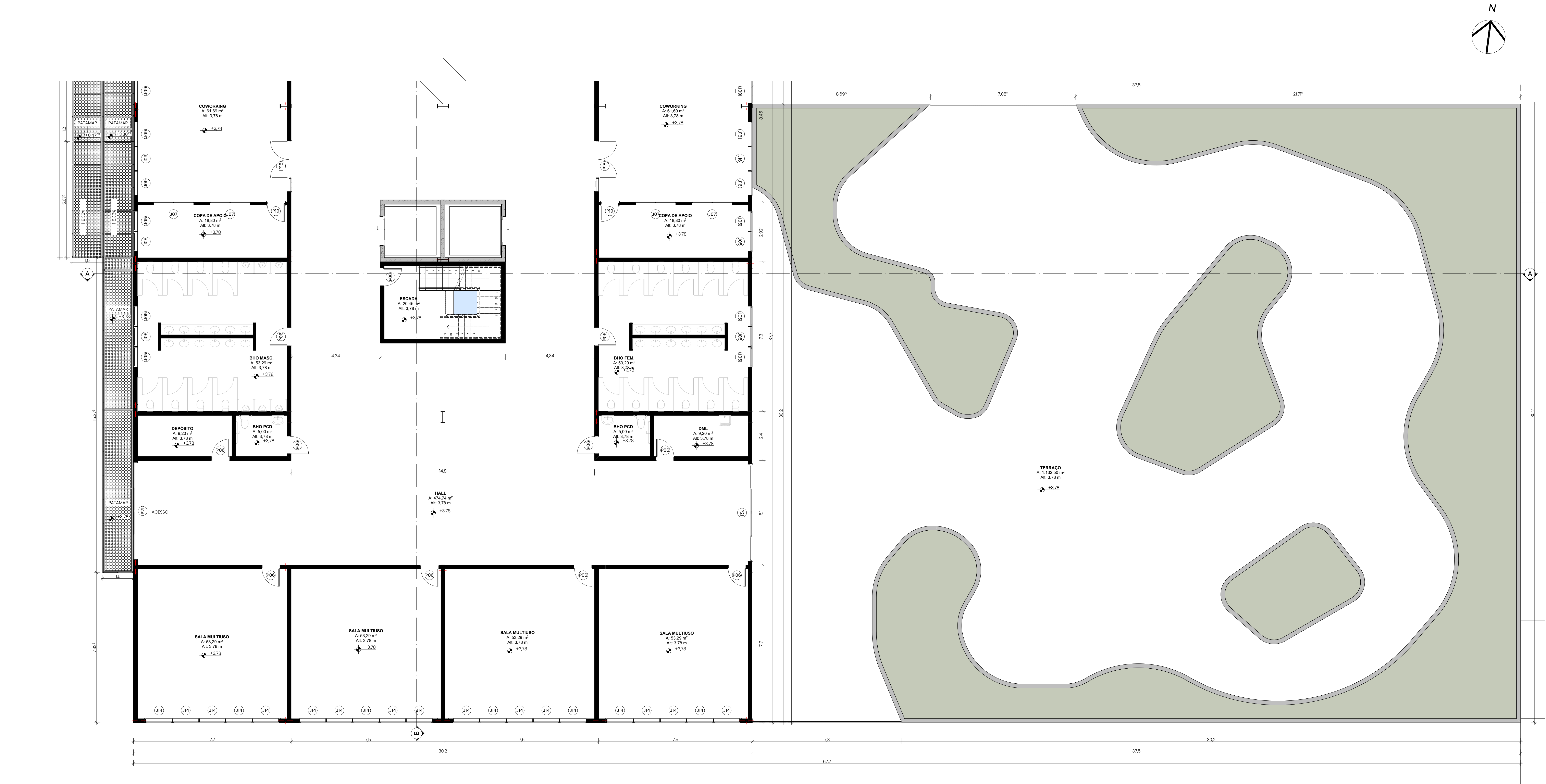
Planta Baixa - Segundo Pavimento 1:75
