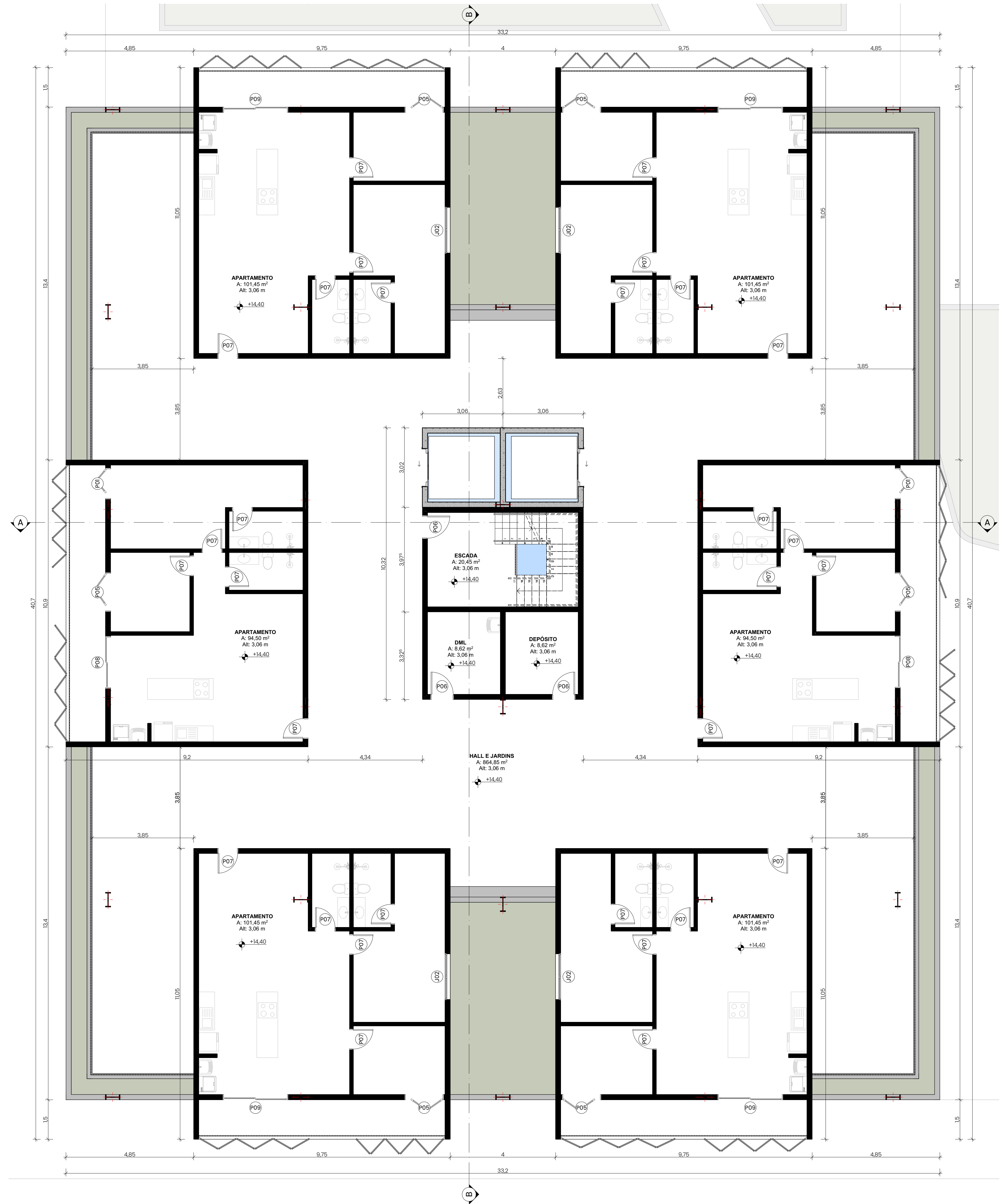
Planta Baixa - Quinto Pavimento (Pav. Tipo 2)
