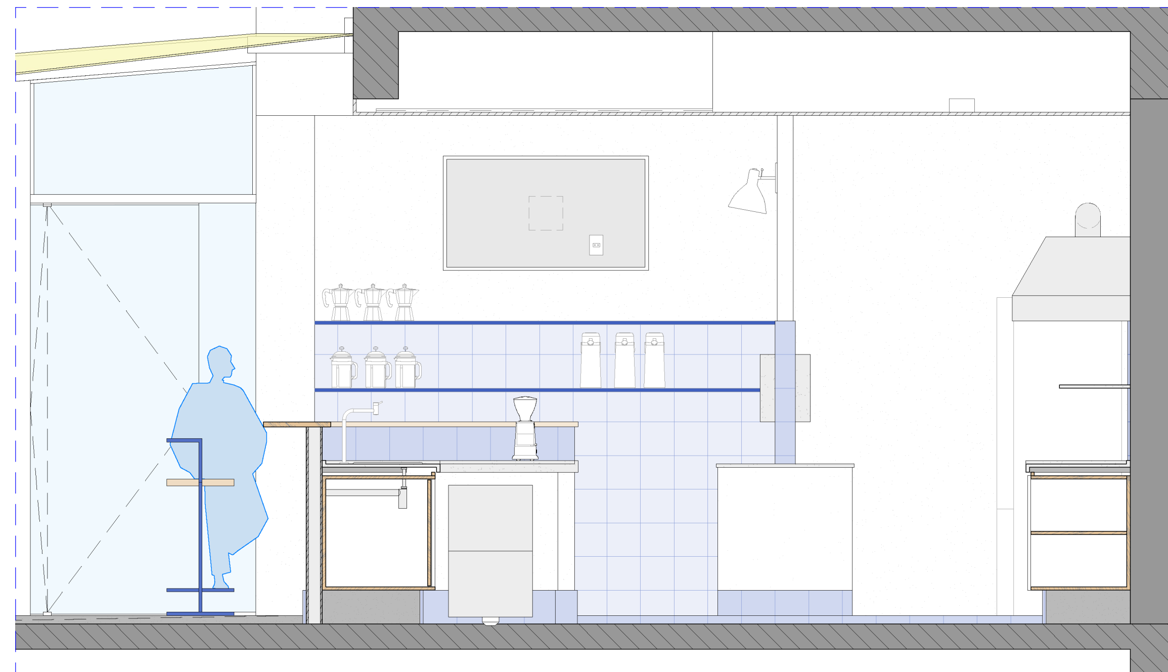
CORTE F
