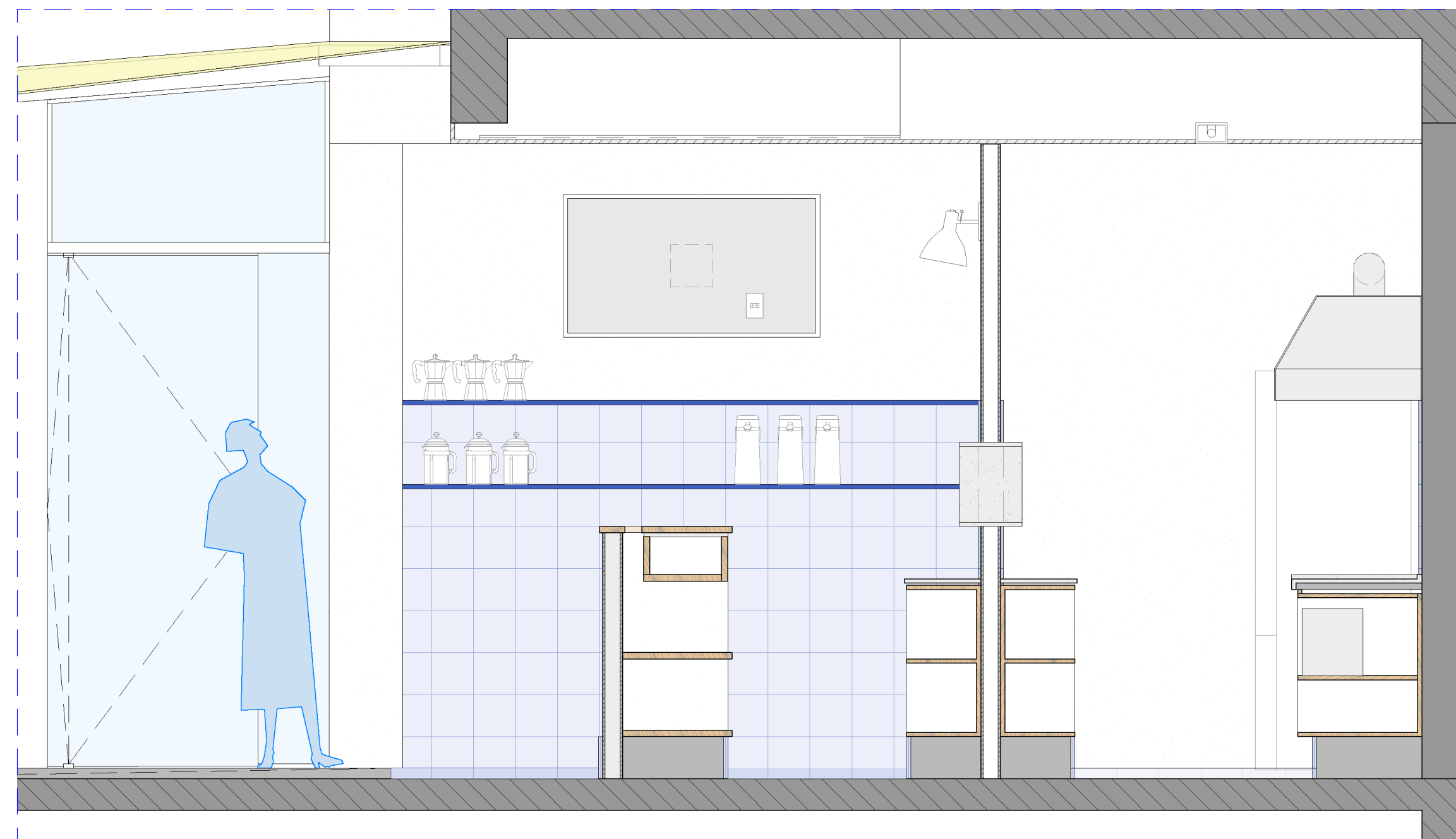
CORTE D
