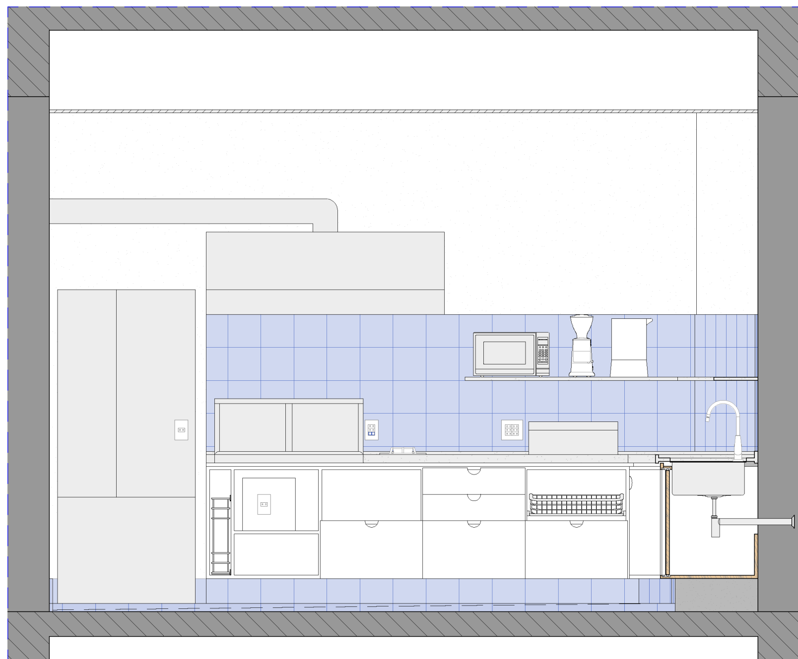
CORTE C
