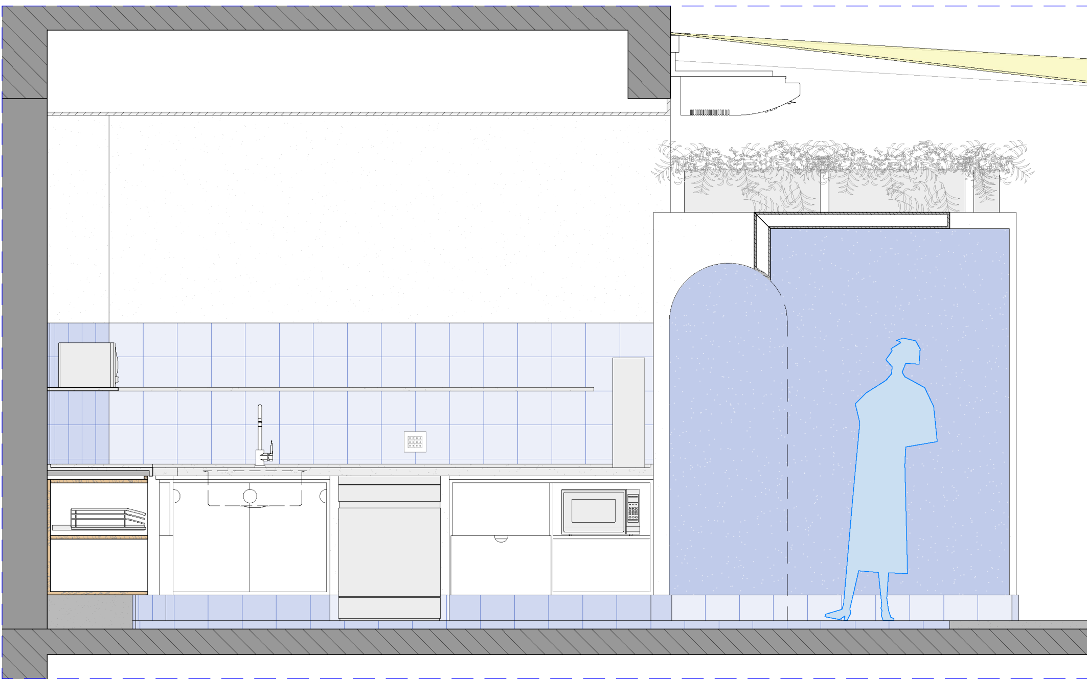
CORTE B
