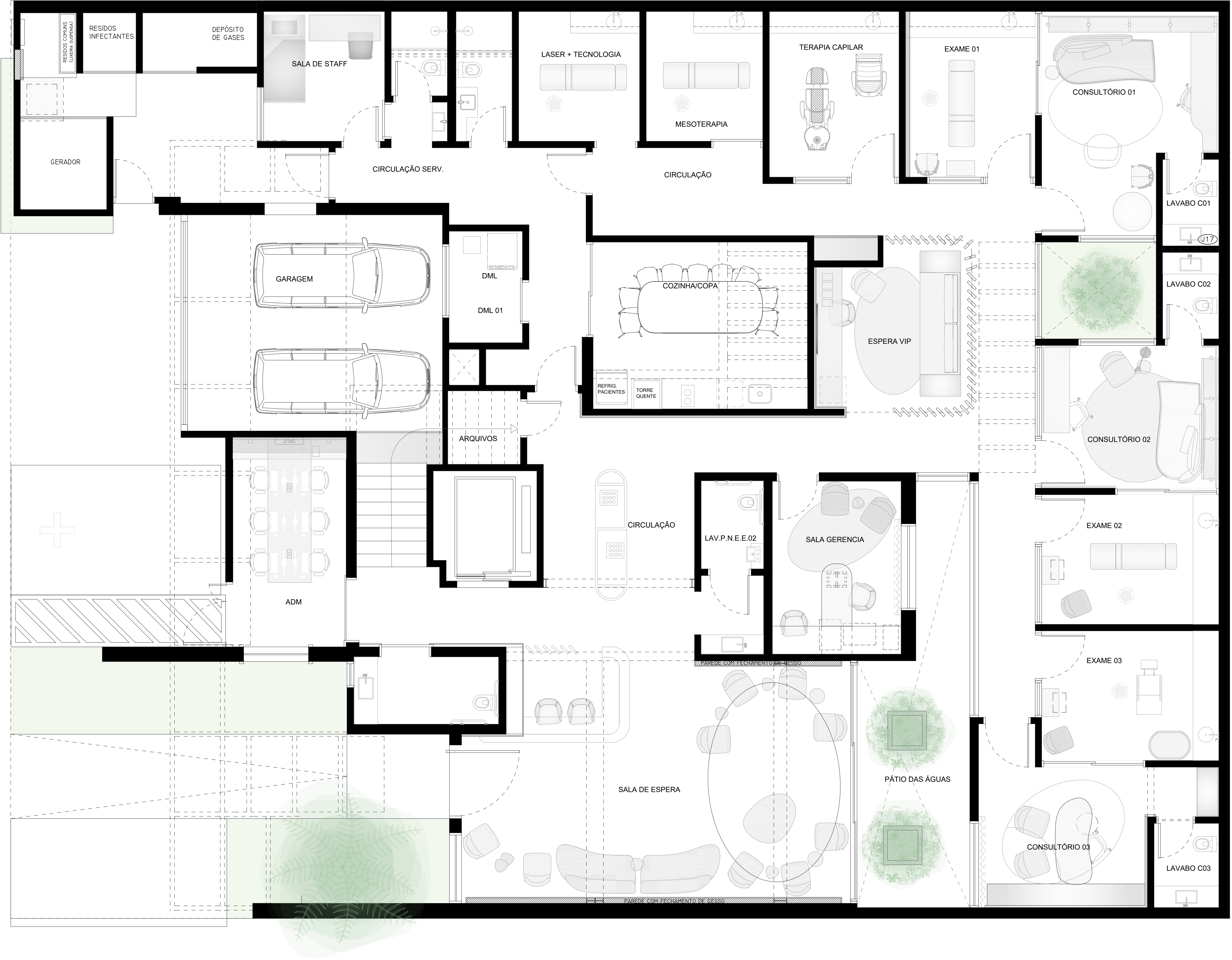
PLANTA BAIXA - PAVIMENTO TÉRREO
