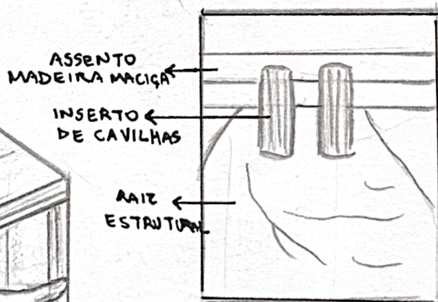
DETALHE A FIXAÇÃO DA RAIZ
