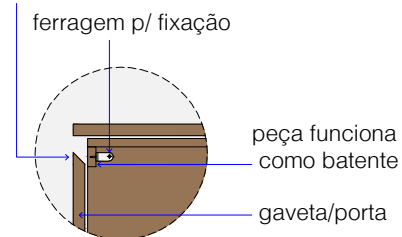
det. puxador cava
