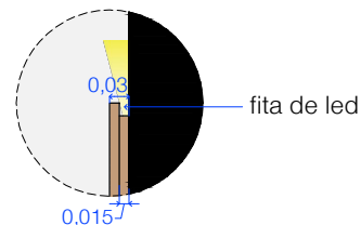
det. painel iluminado
