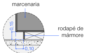
det. genérico rodapé
