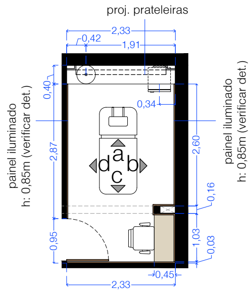
planta sala III
