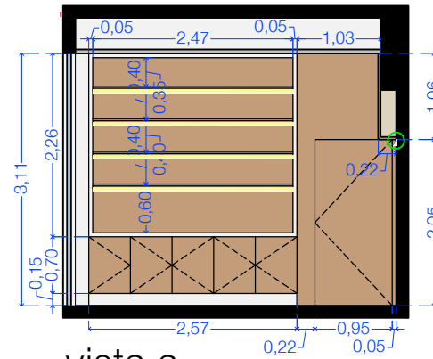
vista a
