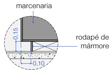
det. genérico rodapé sem escala
