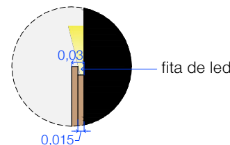
det. painel iluminado sem escala
