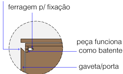
det. puxador cava sem escala
