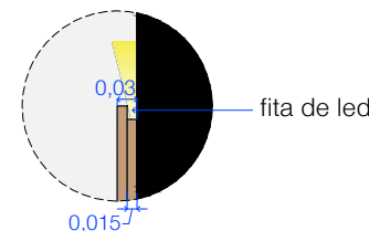
det. painel iluminado sem escala
